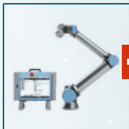
UR10 Roboter E-Serie 6-achsiger Roboter incl. Steuerung und Roboterbedienpanel + schweißtechnische elektr. Entkopplung
